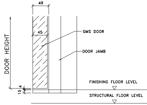
JAMB BOTTOM DETAIL
