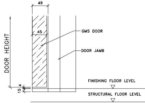
JAMB BOTTOM DETAIL
